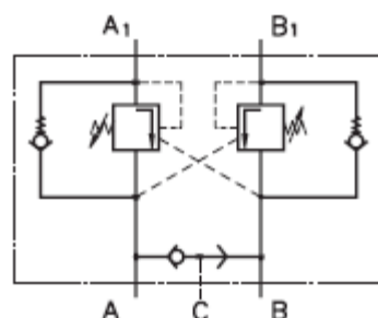
Doppeltwirkendes Senkbremsventil Dual overcenter valve Typ Type KPBT ... D
